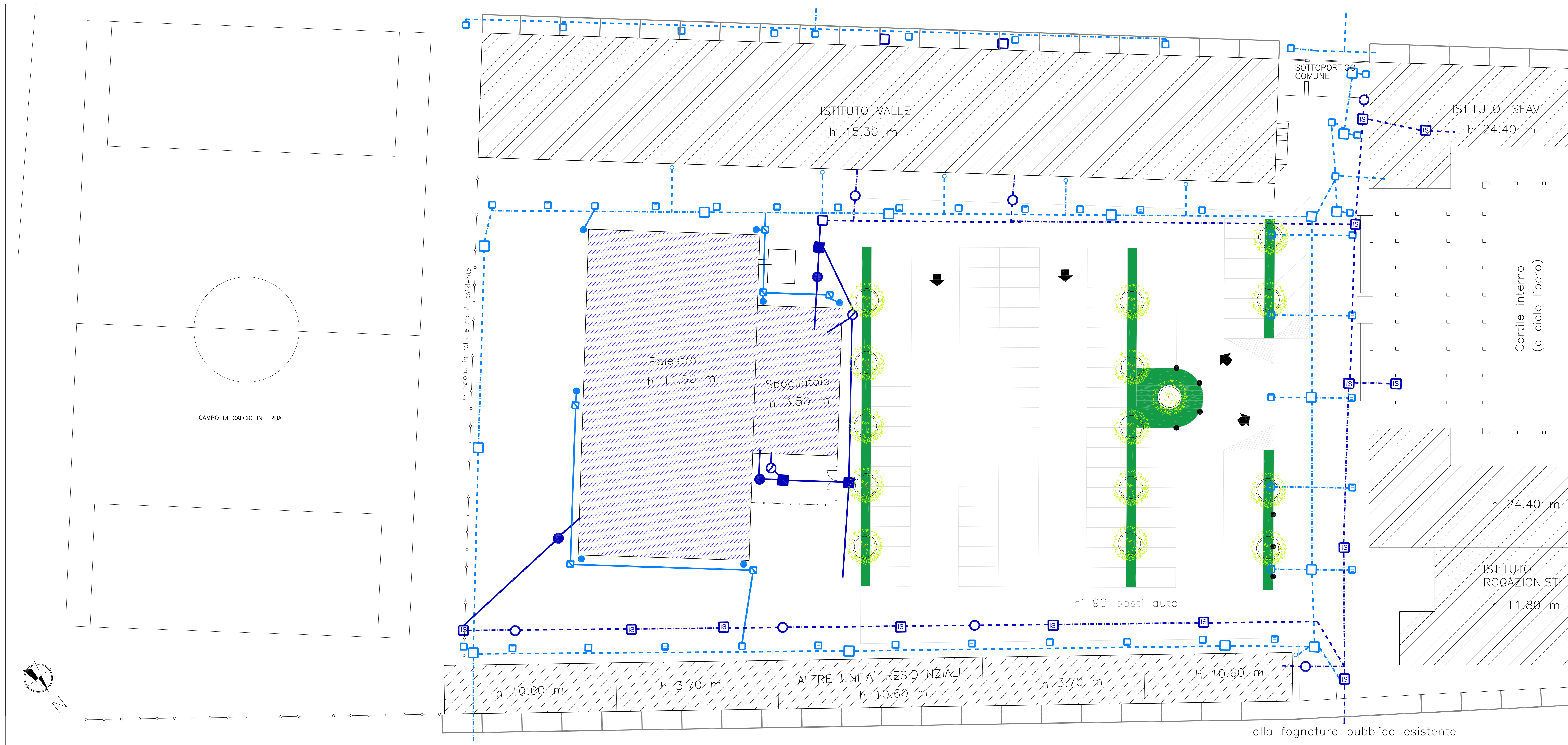
Planimetria - schema linee fognature nere e bianche scala 1:200
