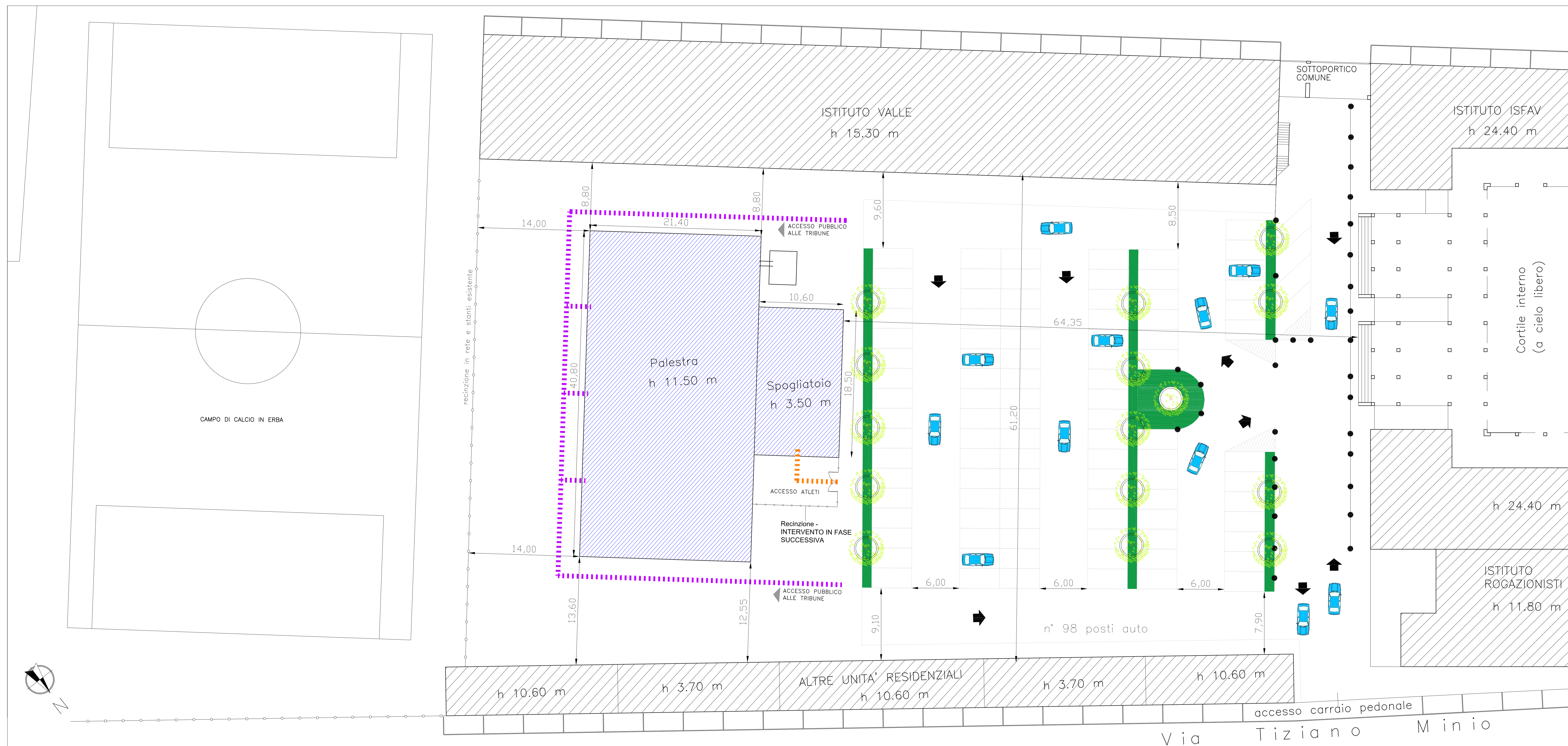
Planimetria Progetto scala 1:200
